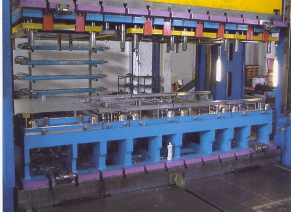
Fig. 3 Lo stampo sotto la pressa
